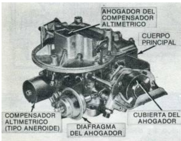
MOTORCRAFT 2150 (vista posterior)
